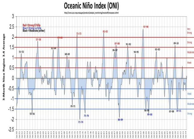
Figure 3.3-9 El Nino/ La Nina index quantified by Niño 3.4 ONI index (NOAA)
